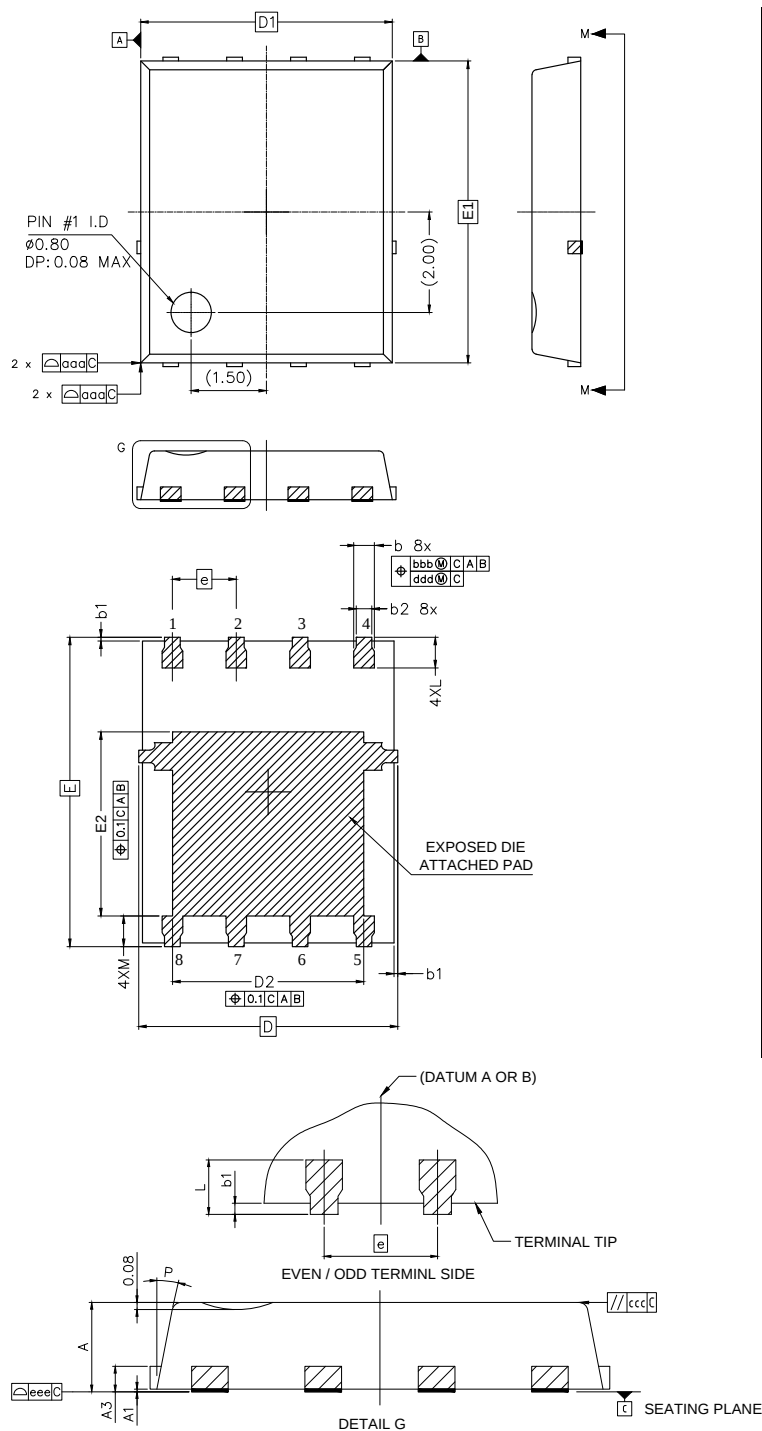
PDFN5x6-8L Package
