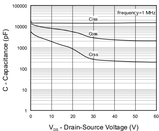
Fig 11. Capacitance
