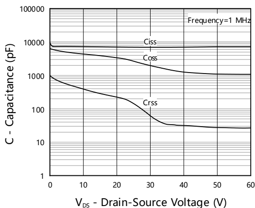
Fig 11. Capacitance
