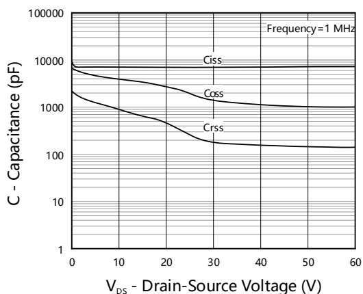
Fig 11. Capacitance
