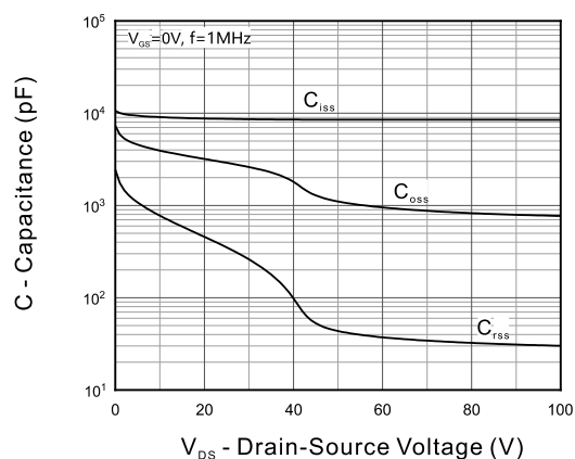
Fig 11. Capacitance
