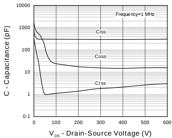
Fig 11. Capacitance
