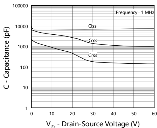
Fig 11. Capacitance
