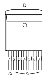
TO-263-7L Plus
