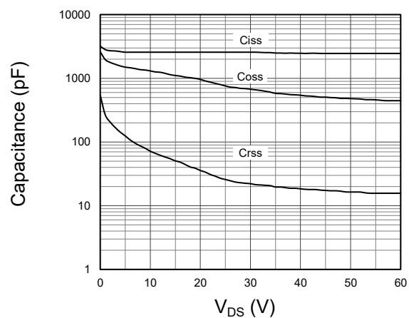
Fig 10. Capacitance
