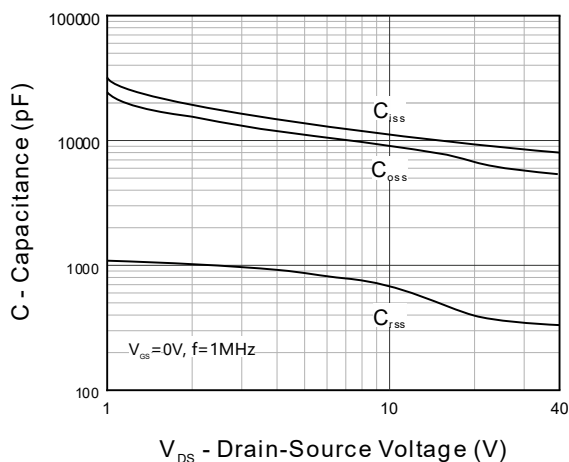
Fig 11. Capacitance
